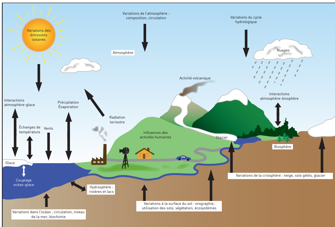
Figure 4 : Représentation des différents compartiments du système climatique et de leurs interactions Source : 4 e rapport du GIEC.
