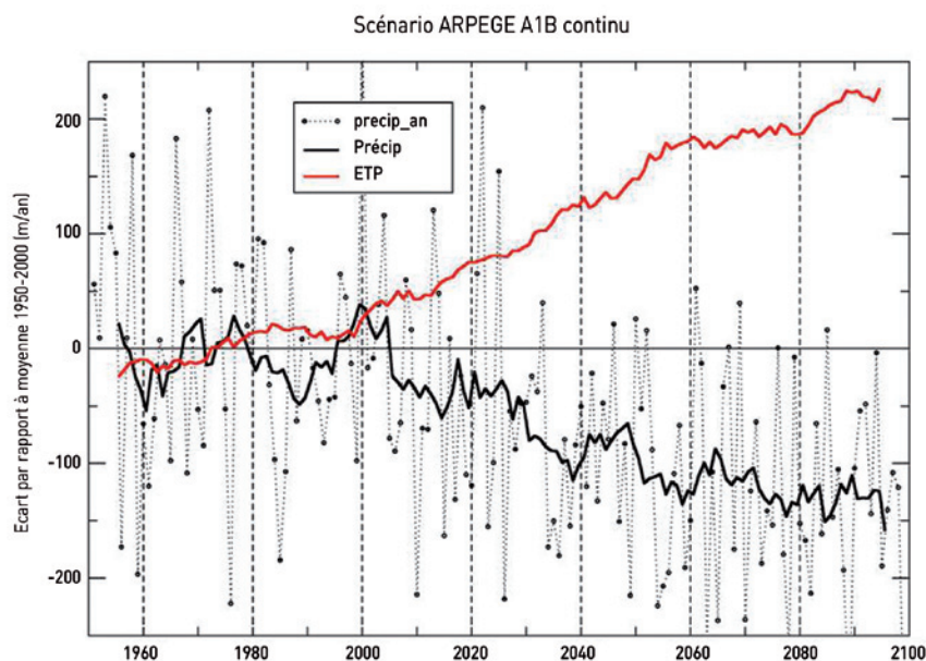
Figure 21 : Évolution des précipitations et de l'évapotranspiration potentielle au cours du XXI e siècle projetée par le modèle ARPEGE sous scénario SRES A1B, désagrégé par la méthode des régimes de temps. Les courbes présentent un lissage sur dix ans, alors que la courbe en pointillés montre la variabilité annuelle des précipitations.
