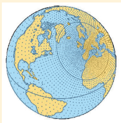
Figure 11 : Maillage irrégulier du modèle ARPEGE. La résolution maximale se situe à proximité de la France.
