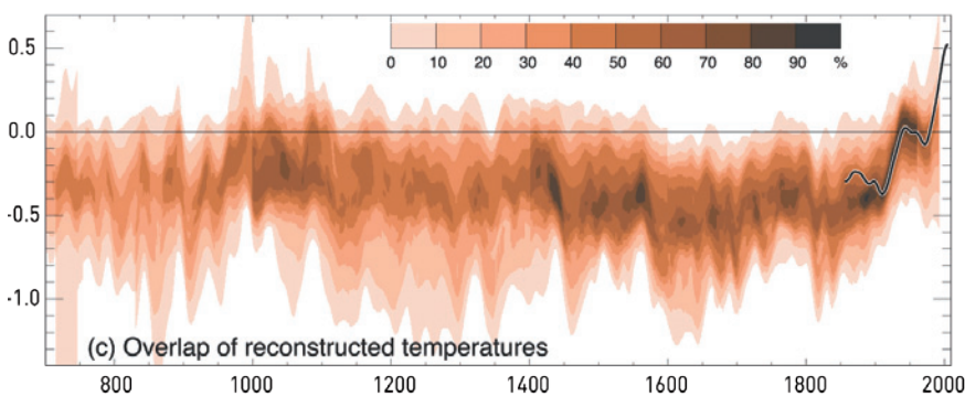
Figure 2 : Évolution de la température de l'air sur les 1 300 dernières années dans l'hémisphère Nord obtenue à partir de plusieurs observations indirectes de la température par rapport à la moyenne sur la période 1961-1990. Source : 4 e rapport du GIEC, chapitre 6.
