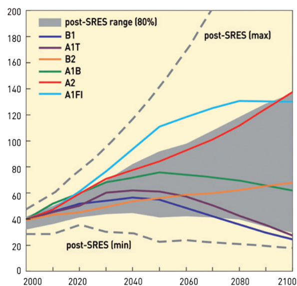
Figure 15 : Émissions mondiales de GES (en gigatonnes équivalent CO 2 par an) en l'absence de politiques climatiques additionnelles.
