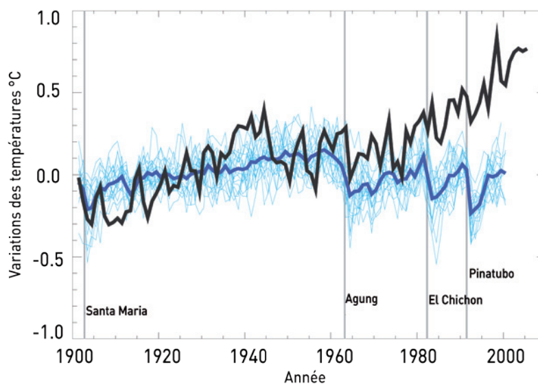
Figure 7 : Variations de la température mondiale moyenne à la surface de la terre sur la période 1901–1950. Par rapport à la figure 6, les variations simulées de la température mondiale moyenne (en bleu) sont basées uniquement sur les concentrations de gaz à effet de serre et d'aérosols d'origine naturelle.
