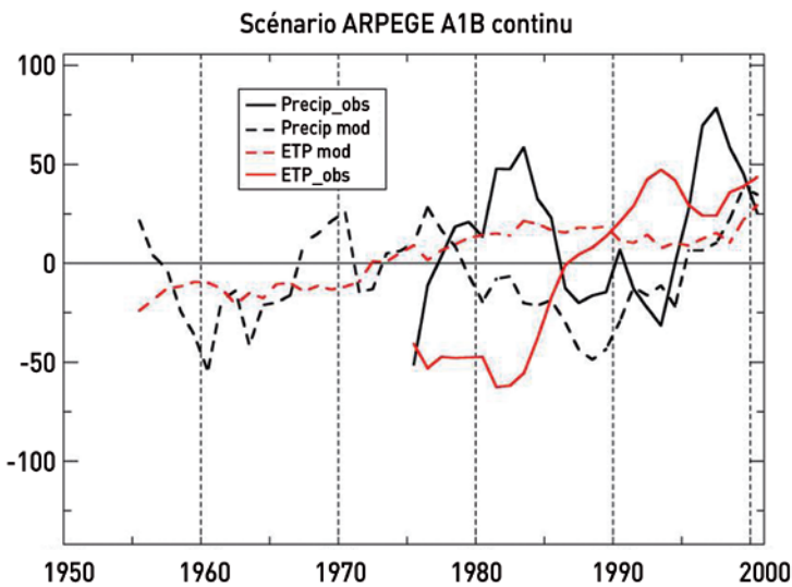
Figure 19 : Évolution des précipitations et de l'évapotranspiration potentielle moyennée par rapport à la moyenne de la période 1970-2000. Les courbes continues correspondent aux observations, alors que les courbes en pointillés correspondent aux scénarios ARPEGE A1B continu désagrégé par la méthode des régimes de temps.
