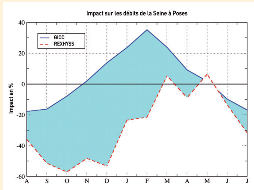
Figure 31 : Comparaison des impacts du changement climatique sur le bassin de la Seine à Poses obtenus lors de la précédente étude GICC, et ceux obtenus lors du projet RExHySS.
