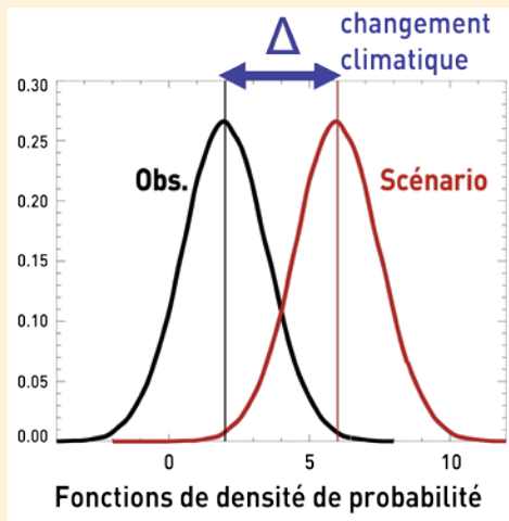
Figure 12 : Principe de la méthode des anomalies. La projection du climat dans le futur conserve la distribution des valeurs observées dans le temps présent, mais reste décalée par une perturbation déduite des simulations climatiques en temps futur et en temps présent. Source : étude de Boé 2007.
