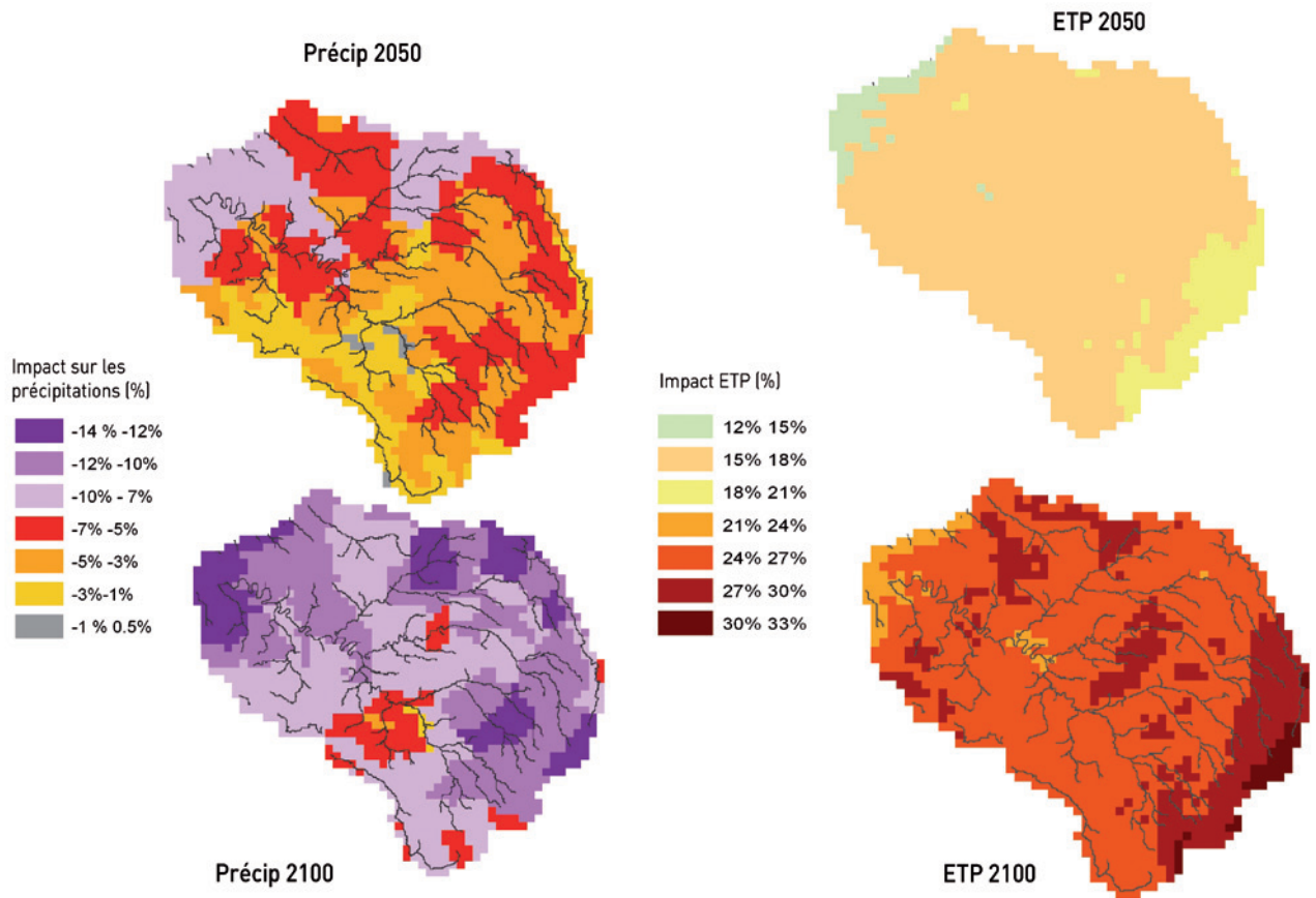
Figure 22 : Moyenne des évolutions par rapport au temps présent des précipitations et de l'ETP à l'horizon 2050 et 2100, estimée par les modèles de climat sous scénario A1B désagrégés par la méthode des régimes de temps.
