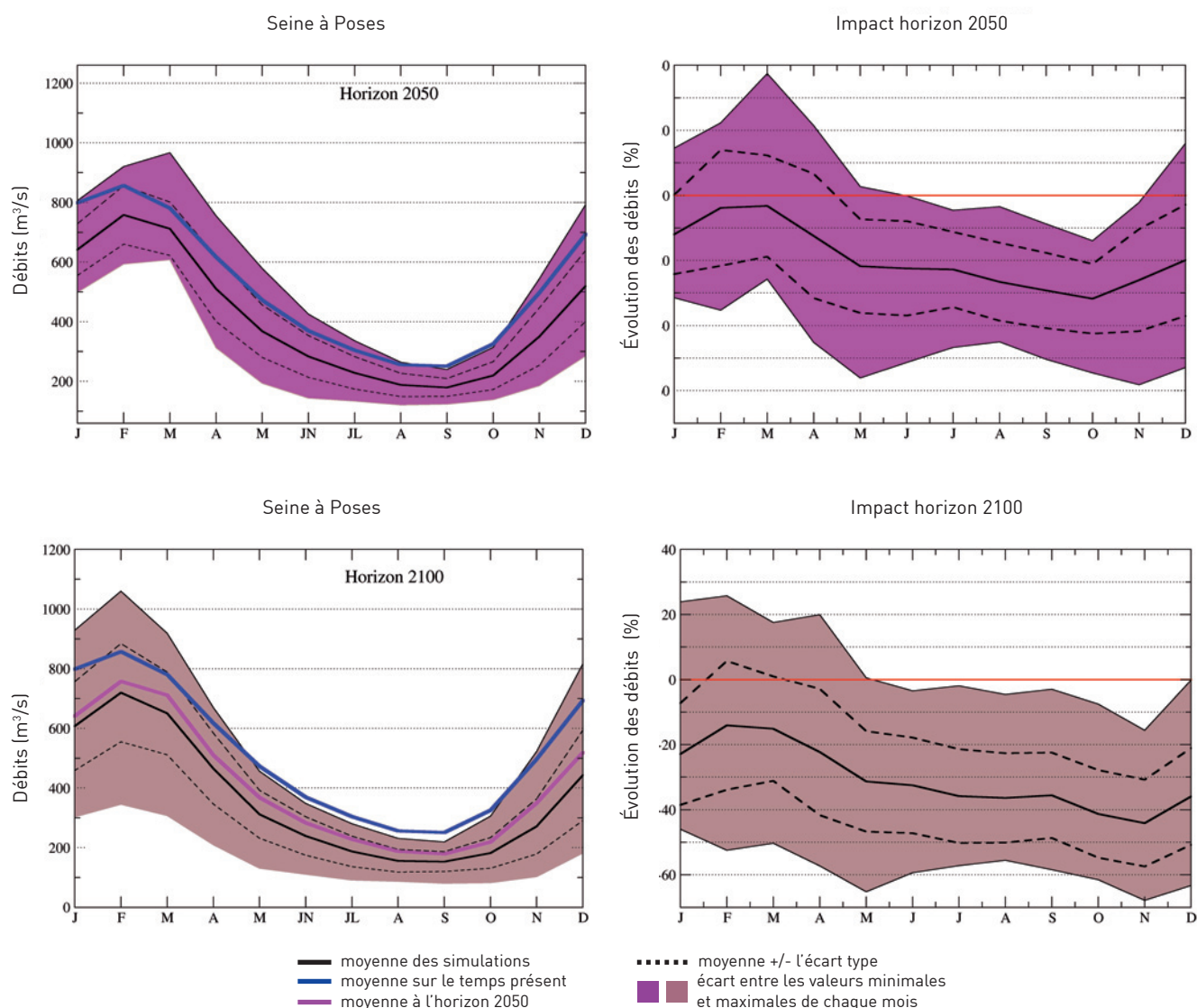
Figure 27 : Impact du changement climatique sur les débits de la Seine à Poses aux horizons 2050 et 2100.
