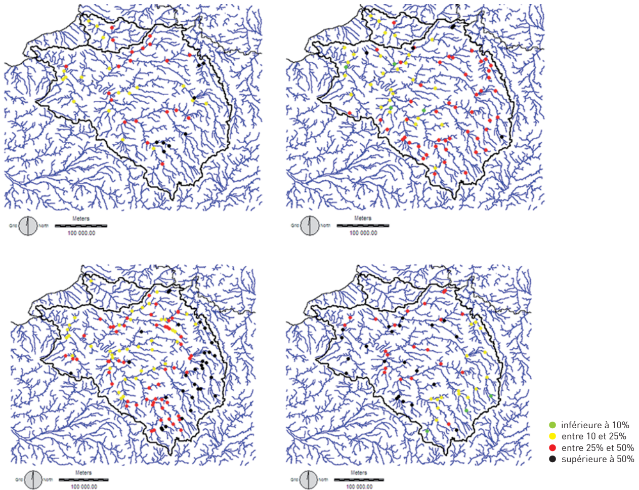
Figure 28 : Cartes des évolutions du QMNA5 (débits représentatifs des étiages) en relatif par rapport aux valeurs temps présent pour les scénarios A1B Milieu de siècle, simulées, de droite à gauche et de haut en bas par EROS, GR4J, MODCOU et SIM. Chaque point représente une station hydrométrique.
