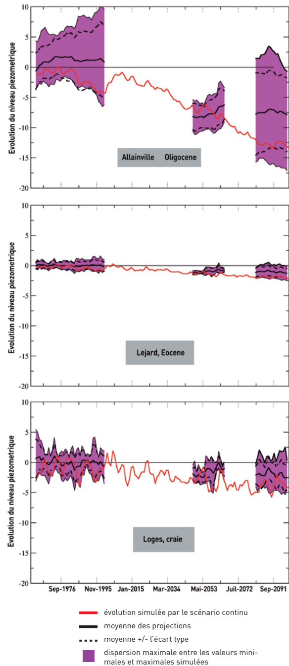
Figure 29 : Évolution du niveau piézométrique de trois stations présentant des variations sensiblement différentes par rapport à la moyenne de référence temps présent.
