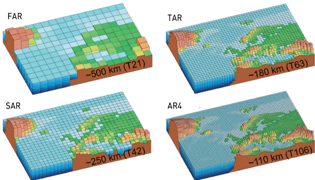
Figure 8 : Relief d'une partie étendue de l'Europe tel qu'il est vu par les modèles de climat pour différentes résolutions spatiales. Les modèles de climat ayant participé au 4 e rapport du GIEC ont des résolutions de l'ordre de 300 km, mais, les plus fins pouvaient avoir une résolution de 110 km de côté. Source : 4 e rapport du GIEC.
