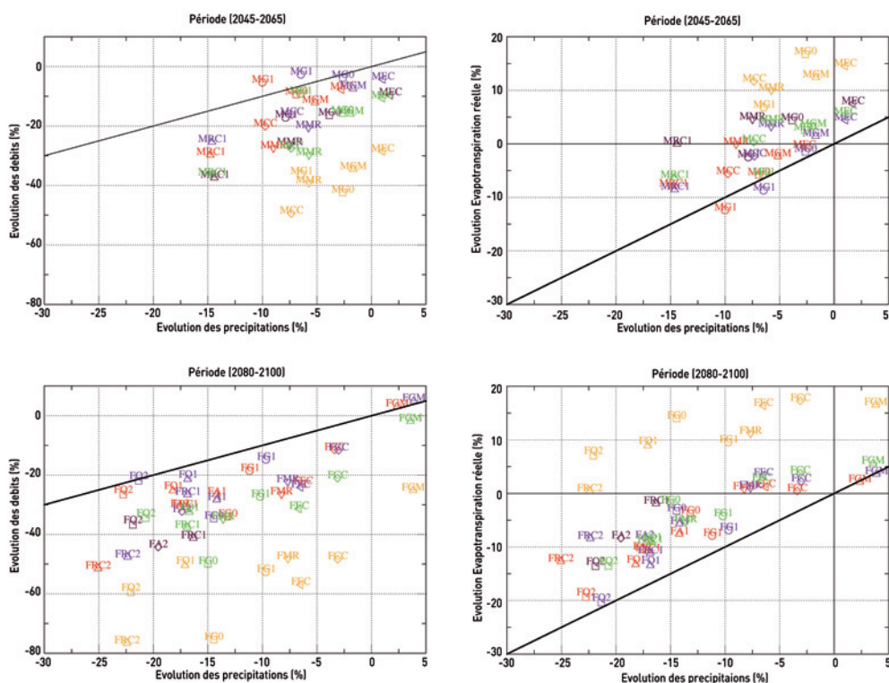
Figure 24 : Représentation de l'évolution de l'évaporation réelle et des débits en fonction de l'évolution des précipitations à l'horizon 2050 et 2100. Chaque symbole correspond à une simulation, les lettres correspondent à une projection climatique désagrégée, et les couleurs aux différents modèles hydrologiques. La courbe 1 : 1 pour laquelle les évolutions des deux variables sont identiques est tracée en ligne épaisse.
