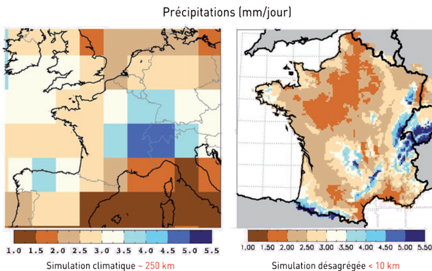
Figure 9 : Illustration de l'impact de la désagrégation. La désagrégation (par la méthode des régimes de temps) permet de retrouver les fortes précipitations sur les zones de relief (Pyrénées, Alpes, Cévennes, Massif Central, Vosges et Jura).
