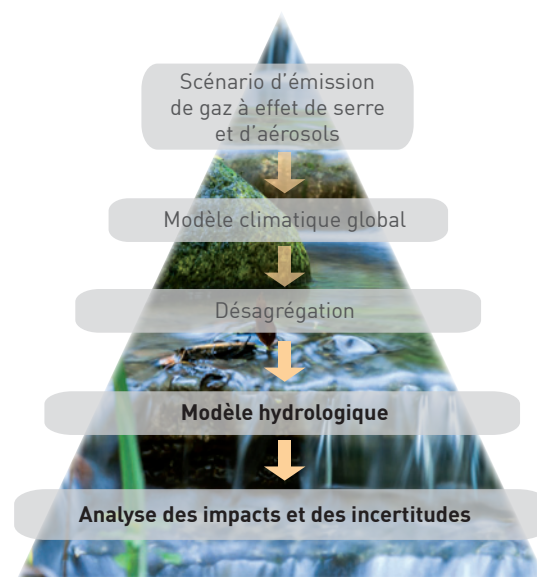
Figure 23 : Situation par rapport à la méthodologie générale.
