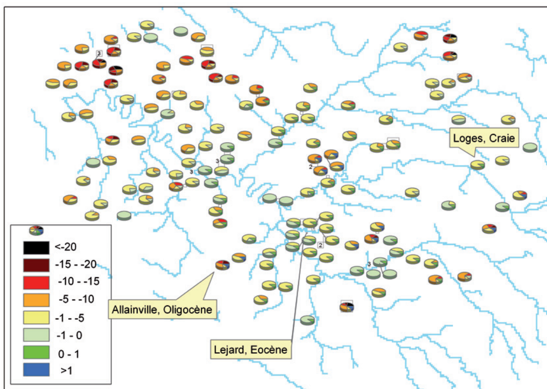
Figure 30 : Impact du changement climatique sur 137 piézomètres tel que simulés par MODCOU avec 9 projections climatiques désagrégées. Les camemberts montrent l'évolution des piézométries en mètre sur les 9 projections : en haut, horizon 2050 et en bas, horizon 2100.
