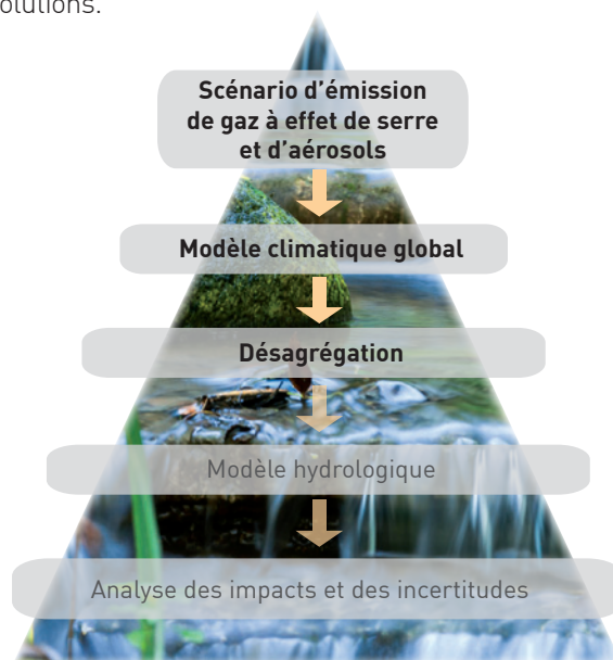
Figure 17 : Situation par rapport à la méthodologie générale. Les éléments en gras sont impliqués dans ce chapitre.
