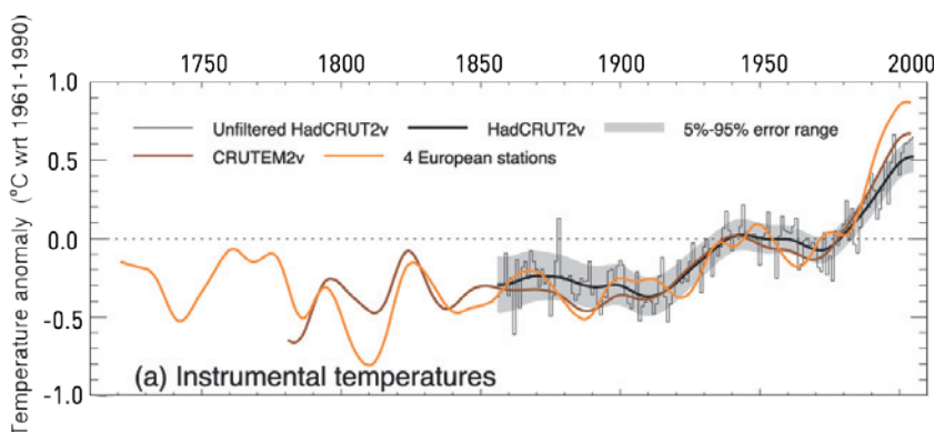
Figure 3 : Détails de la figure précédente sur les 250 dernières années, intégrant en complément différentes estimations basées sur des observations de température. Source : 4 e rapport du GIEC.
