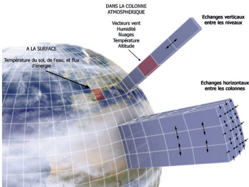
Figure 5 : Principe du découpage en maille utilisé par les modèles atmosphériques. Les mailles recouvrent l'ensemble du globe, avec plusieurs niveaux pour représenter les couches atmosphériques. Les échanges entre les mailles peuvent être latéraux ou verticaux.
