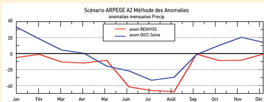
Figure 32 : Impact du changement climatique sur les précipitations mensuelles (en pourcentage d'évolution par rapport au temps présent) obtenus par le modèle ARPEGE sous scénario A2 à l'époque du GICC-Seine (en bleu) et de REXHYSS (en rouge)
