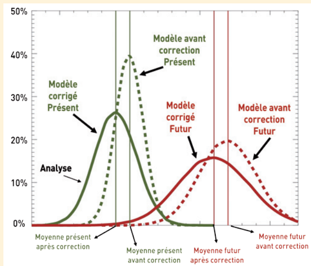
Figure 13 : Principe de la méthode quantile-quantile. On se base sur les distributions observées et simulées en temps présent pour construire une règle de correction. Cette règle est ensuite appliquée sur les simulations climatiques dans le futur pour bâtir une projection futur corrigée.
