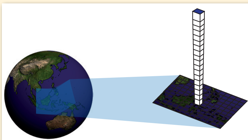
Figure 10 : Principe d'un modèle régional qui utilise les simulations d'un modèle global pour définir les conditions aux limites. Ce modèle simule, sur un domaine limité, l'ensemble des circulations atmosphériques en 3D. Le domaine plus réduit permet de raffiner la résolution spatiale.
