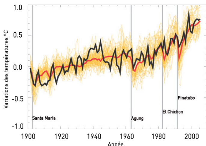
Figure 6 : Variations de la température mondiale moyenne à la surface de la terre par rapport à la période 1901-1950, telles qu'elles ont été observées et telles qu'elles ont été simulées par des modèles climatiques prenant en compte les concentrations en gaz à effet de serre et en aérosols d'origine naturelle et anthropique. Les lignes grises verticales indiquent les dates d'événements volcaniques majeurs, qui en augmentant la quantité d'aérosols dans l'atmosphère ont un impact sur le climat.
