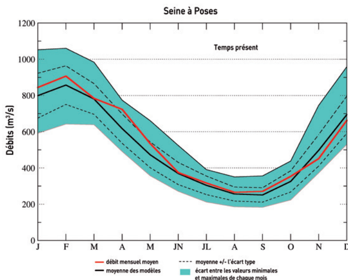
Figure 26 : Débits mensuels moyens simulés par les modèles hydrologiques utilisant les simulations temps présents des modèles climatiques désagrégés.
