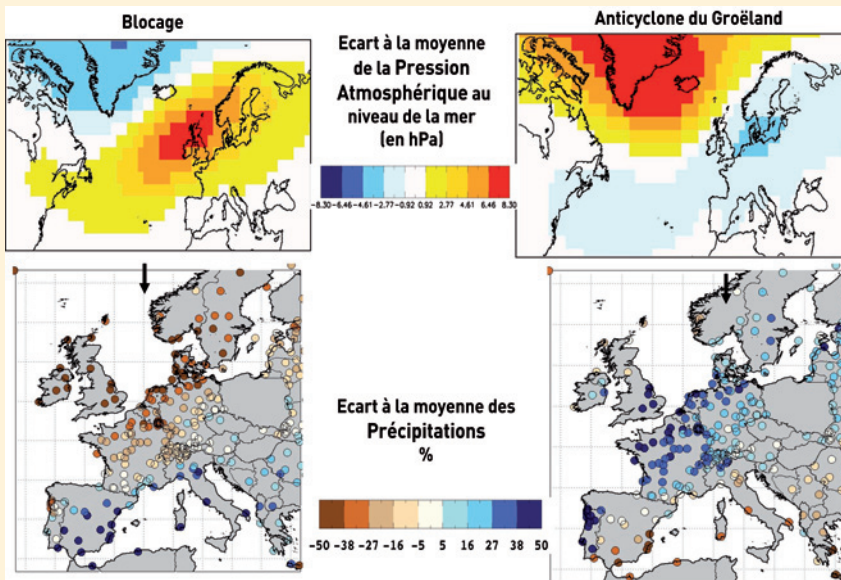
Figure 14 : Illustration du lien entre un « prédicteur » de grande échelle et des caractéristiques locales sur deux situations observées contrastées. En haut, des écarts à la moyenne de la pression atmosphérique au niveau de la mer, présentant un anticyclone situé sur l'Irlande à gauche, et sur le Groënland à droite, et en bas, caractéristique des précipitations associées à ces deux types de temps : à gauche, on constate une tendance à de faibles précipitations sur le nord de la France, alors qu'à droite, les précipitations sont relativement intenses.
