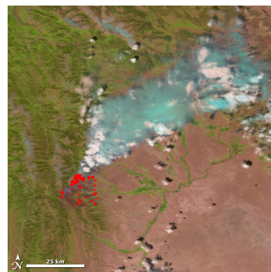
Acquisition de l'instrument VIIRS lors de feux de Wyoming du 1 er Juillet 2012. Les foyers rouges représentent les zones actives des feux.
