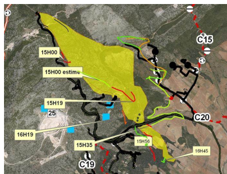
Synthèse du REX66 lors du feu de Vin-grau (09/08/2011).
