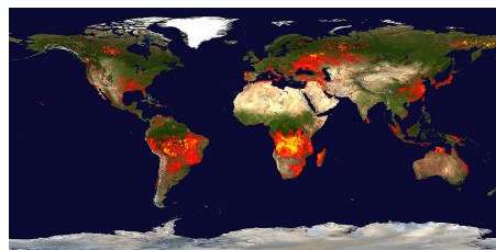
Carte mondiale de synthèse MODIS de la localisation des feux de forêts pour la période du 30 Juillet au 8 Août 2010.
