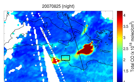
Acquisition de l'instrument IASI (monoxyde de carbone) lors de feux de Grèce de 2007.
