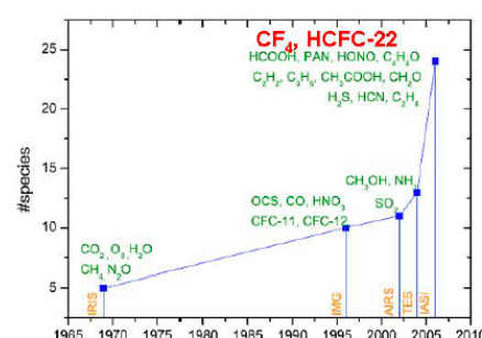
Évolution du nombre d'espèces chimiques mesuré par interférométrie spatiale au cours du temps.
