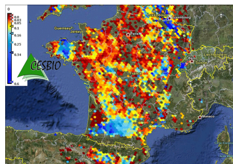
Acquisition de l'instrument SMOS (humidité des sols) lors de la sécheresse de 2010.
