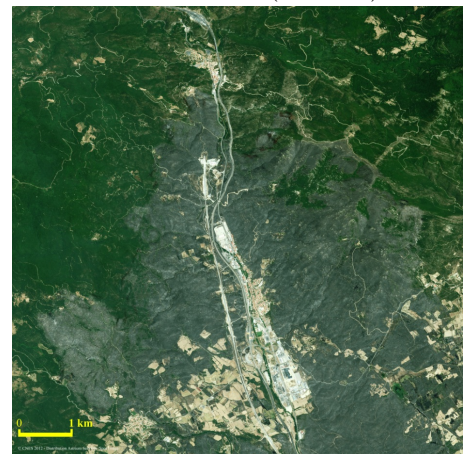
Image PLEIADES de la zone brûlée par le feu du Perthus du 24 Juillet 2012 (©Astrium).
