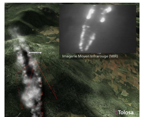
Principe d'une acquisition LiveFire dans le moyen infrarouge (©iTolosa).
