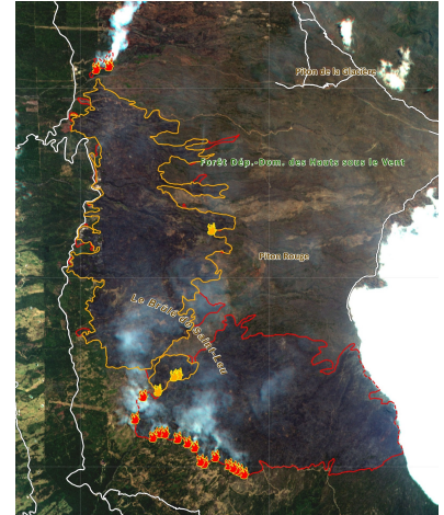
Image traitée des feux de la Réunion de 2011 (©SERTIT).
