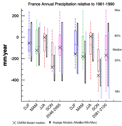
FIG. 10: Diagramme en boîte de l'anomalie de précipitations pour les périodes 2046-2065 et 2081-2100 avec comme période de référence 1961-1990. Les boîtes de couleurs représentent la moyenne des simulation GIEC, les noires représentent les 4 simulations ARPEGE V4 CERFACS, et les boîtes violettes représentent les 3 simulations ARPEGE V4 RETIC. Le symbole X présente la simulation du modèle CNRM-CM3 de Météo-France. Les boîtes noires et violettes ne présentent que les extrêmes maximum et minimum de même que la médiane (pas de lignes tiretées). La moyenne spatiale est calculée sur un domaine couvrant la France entière.
