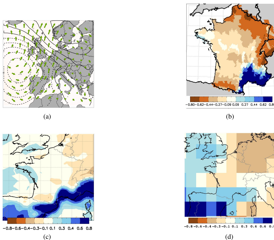
FIG. 2: (a) présente un régime de temps présentant un flux de vent du sud sur la France. Les vents à 850 hPa sont présentés sous forme de vecteurs, l'anomalie de pression au niveau moyen de la mer en lignes noires (tiretées pour les valeurs négatives). Associées à ce régime de temps, anomalie de précipitations (%) observée en (b), telle que simulée par un modèle régional du climat en (c), et telle que simulée par un modèle global du climat en (d).
