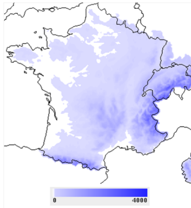
FIG. 3: Analyse météorologique à méso-échelle de Météo-France : SAFRAN. L'altitude de chacun des points de l'analyse est présentée. La résolution spatiale est de 8 km, en grille régulière sur une projection Lambert-II étendue.
