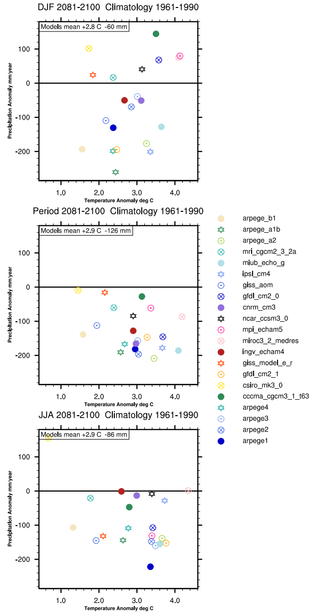
FIG. 6: Graphiques \Delta T \Delta P présentant les anomalies de température et précipitation pour l'hiver DJF (en haut), l'été JJA (en bas), et la moyenne annuelle (au centre). La période présentée est 2081-2100 avec comme référence 1961-1990, la moyenne spatiale étant calculée sur un domaine couvrant la France entière.
