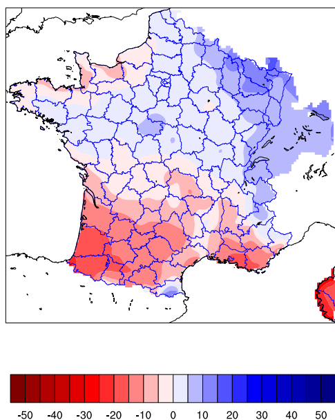
FIG. 11: Moyenne multi-modèles des anomalies de précipitation (mm/an) pour la période hivernale (décembre-janvier-février (DJF)) de la période 2046-2065 par rapport à la climatologie 1961-1990. Les modèles sont ceux du GIEC ainsi que les 7 simulations ARPEGE V4.
