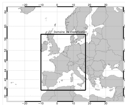
FIG. 4: Domaine de grande échelle utilisé (rectangle noir).
