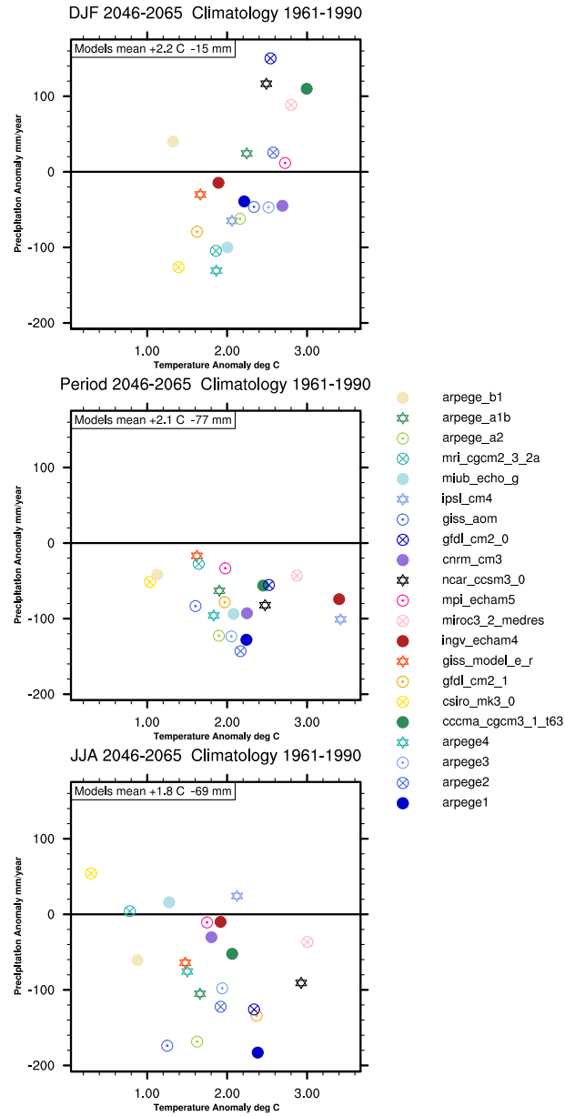
FIG. 5: Graphiques \Delta T \Delta P présentant les anomalies de température et précipitation pour l'hiver DJF (en haut), l'été JJA (en bas), et la moyenne annuelle (au centre). La période présentée est 2046-2065 avec comme référence 1961-1990, la moyenne spatiale étant calculée sur un domaine couvrant la France entière.
