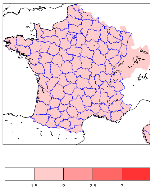
FIG. 14: Moyenne multi-modèles des anomalies de température (degrés C) pour la période estivale (juin-juillet-août (JJA)) couvrant 2046-2065 par rapport à la climatologie 1961-1990. Les modèles sont ceux du GIEC ainsi que les 7 simulations ARPEGE V4.
