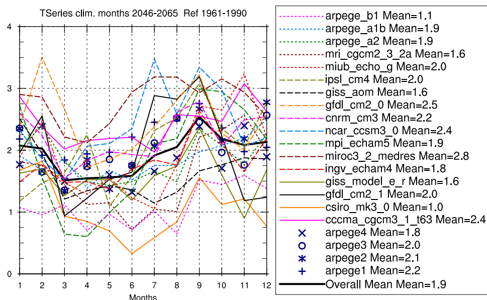
FIG. 7: Anomalies de température moyennées sur chacun des mois (janvier=1 ; décembre=12) de la période 2046-2065 avec comme référence 1961-1990, la moyenne spatiale étant calculée sur un domaine couvrant la France entière.
