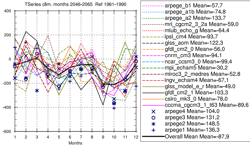
FIG. 8: Anomalies de précipitation moyennées sur chacun des mois (janvier=1 ; décembre=12) de la période 2046-2065 avec comme référence 1961-1990, la moyenne spatiale étant calculée sur un domaine couvrant la France entière.
