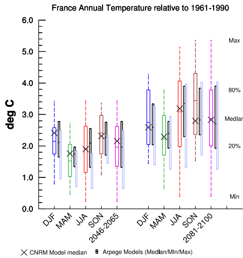
FIG. 9: Diagramme en boîte de l'anomalie de température pour les périodes 2046-2065 et 2081-2100 avec comme période de référence 1961-1990. Les boîtes de couleurs représentent la moyenne des simulation GIEC, les noires représentent les 4 simulations ARPEGE V4 CERFACS, et les boîtes violettes représentent les 3 simulations ARPEGE V4 RETIC. Le symbole X présente la simulation du modèle CNRM-CM3 de Météo-France. Les boîtes noires et violettes ne présentent que les extrêmes maximum et minimum de même que la médiane (pas de lignes tiretées). La moyenne spatiale est calculée sur un domaine couvrant la France entière.
