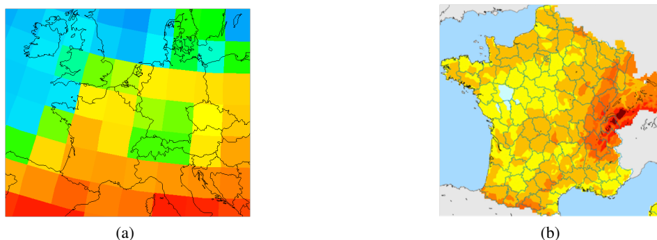
FIG. 1: Exemple de données de précipitations (mm/jour) couvrant la France. La figure (a) montre les données à la résolution typique d'un modèle global du climat (modèle IPSL CM4 IPCC-AR4 2.5° x 3.75°), tandis que la figure (b) montre les données désagrégées statistiquement à une résolution de 8 km.
