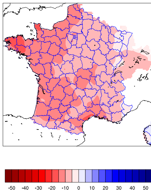
FIG. 12: Moyenne multi-modèles des anomalies de précipitation (mm/an) pour la période estivale (juin-juillet-août (JJA)) couvrant 2046-2065 par rapport à la climatologie 1961-1990. Les modèles sont ceux du GIEC ainsi que les 7 simulations ARPEGE V4.
