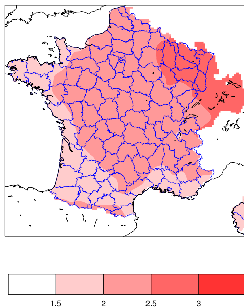
FIG. 13: Moyenne multi-modèles des anomalies de température (degrés C) pour la période hivernale (décembre-janvier-février (DJF)) couvrant 2046-2065 par rapport à la climatologie 1961-1990. Les modèles sont ceux du GIEC ainsi que les 7 simulations ARPEGE V4.
