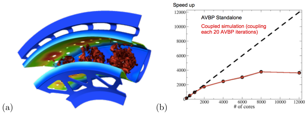
FIGURE 4 – Couplage SGE réactive couplée au calcul thermique solide pour une chambre de combustion aéronautique : (a) vue de la géométrie avec les trois flammes présentes devant chaque système d’injection, accompagnée du champ de température de paroi issu du code de thermique du solide et (b) courbe de scalabilité du problème couplé.
