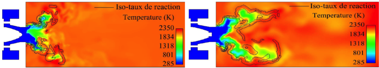
FIGURE 3 – Configuration MERCATO (ONERA) : champ de température. Gauche : résultat Lagrangien ; Droite : résultat Eulérien.
