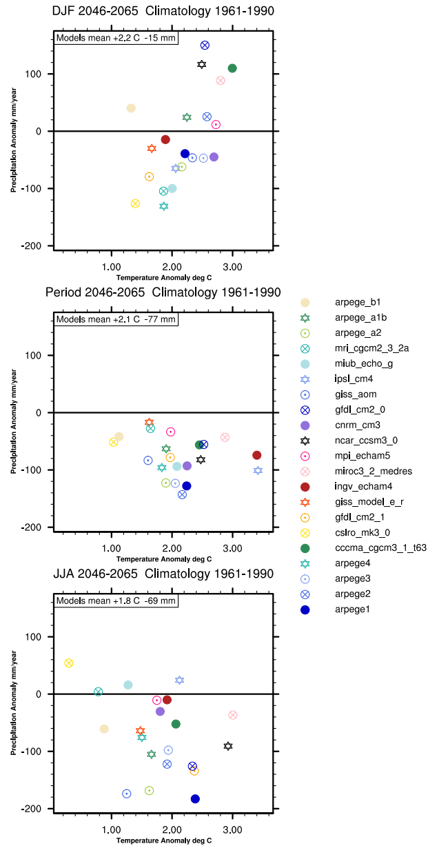
FIGURE 5 – Graphiques \Delta T \Delta P présentant les anomalies de température et précipitation pour l'hiver DJF (en haut), l'été JJA (en bas), et la moyenne annuelle (au centre). La période présentée est 2046-2065 avec comme référence 1961-1990, la moyenne spatiale étant calculée sur un domaine couvrant la France entière.
