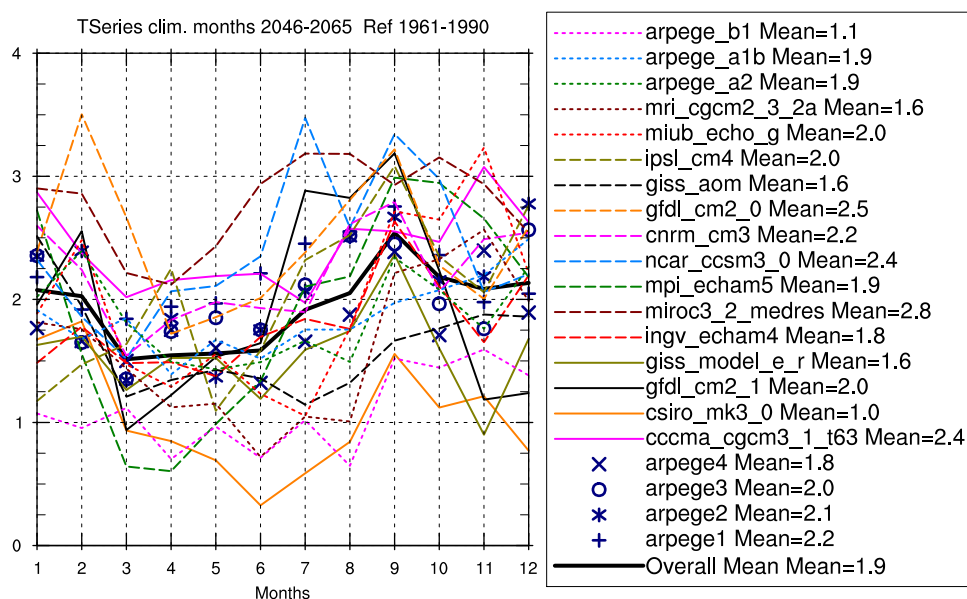
FIGURE 7 – Anomalies de température moyennées sur chacun des mois (janvier=1 ; décembre=12) de la période 2046-2065 avec comme référence 1961-1990, la moyenne spatiale étant calculée sur un domaine couvrant la France entière.
