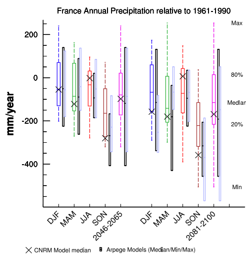
FIGURE 10 – Diagramme en boîte de l’anomalie de précipitations pour les périodes 2046-2065 et 2081-2100 avec comme période de référence 1961-1990. Les boîtes de couleurs représentent la moyenne des simulation GIEC, les noires représentent les 4 simulations ARPEGE V4 CERFACS, et les boîtes violettes représentent les 3 simulations ARPEGE V4 RETIC. Le symbole X présente la simulation du modèle CNRM-CM3 de Météo-France. Les boîtes noires et violettes ne présentent que les extrêmes maximum et minimum de même que la médiane (pas de lignes tiretées). La moyenne spatiale est calculée sur un domaine couvrant la France entière.
