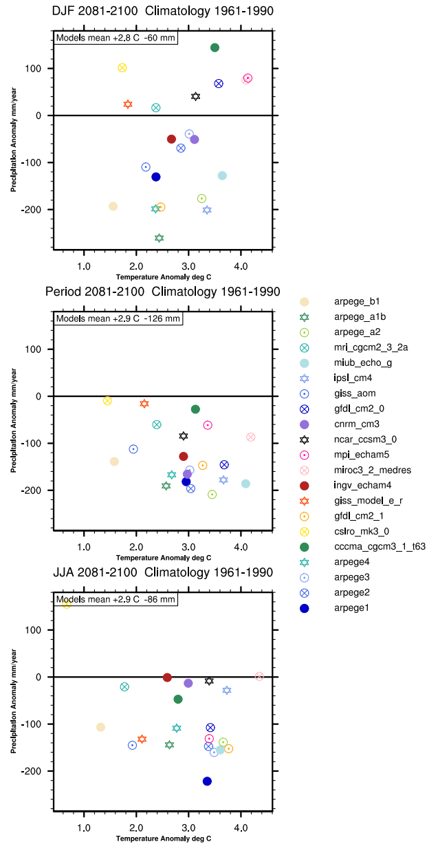
FIGURE 6 – Graphiques \Delta T \Delta P présentant les anomalies de température et précipitation pour l'hiver DJF (en haut), l'été JJA (en bas), et la moyenne annuelle (au centre). La période présentée est 2081-2100 avec comme référence 1961-1990, la moyenne spatiale étant calculée sur un domaine couvrant la France entière.
