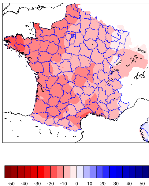
FIGURE 12 – Moyenne multi-modèles des anomalies de précipitation (mm/an) pour la période estivale (juin-juillet-août (JJA)) couvrant 2046-2065 par rapport à la climatologie 1961-1990. Les modèles sont ceux du GIEC ainsi que les 7 simulations ARPEGE V4.
