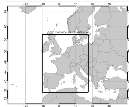
FIGURE 4 – Domaine de grande échelle utilisé (rectangle noir).
