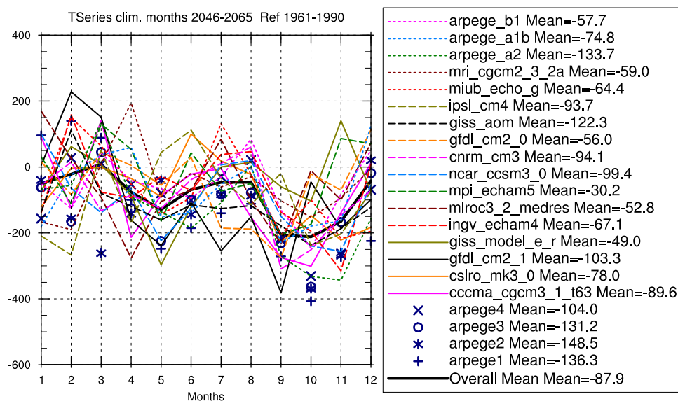
FIGURE 8 – Anomalies de précipitation moyennées sur chacun des mois (janvier=1 ; décembre=12) de la période 2046-2065 avec comme référence 1961-1990, la moyenne spatiale étant calculée sur un domaine couvrant la France entière.
