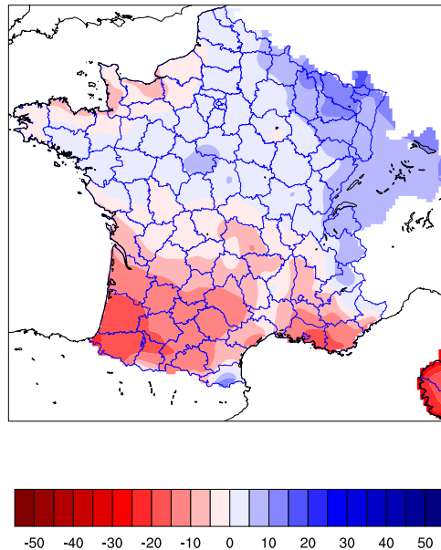
FIGURE 11 – Moyenne multi-modèles des anomalies de précipitation (mm/an) pour la période hivernale (décembre-janvier-février (DJF)) de la période 2046-2065 par rapport à la climatologie 1961-1990. Les modèles sont ceux du GIEC ainsi que les 7 simulations ARPEGE V4.
