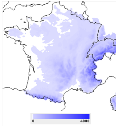
FIGURE 3 – Analyse météorologique à méso-échelle de Météo-France : SAFRAN. L'altitude de chacun des points de l'analyse est présentée. La résolution spatiale est de 8 km, en grille régulière sur une projection Lambert-II étendue.
