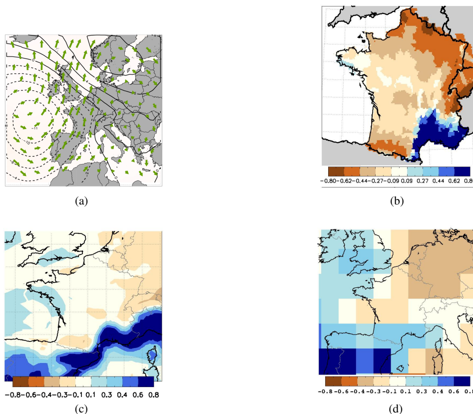
FIGURE 2 – (a) présente un régime de temps présentant un flux de vent du sud sur la France. Les vents à 850 hPa sont présentés sous forme de vecteurs, l'anomalie de pression au niveau moyen de la mer en lignes noires (tiretées pour les valeurs négatives). Associées à ce régime de temps, anomalie de précipitations (%) observée en (b), telle que simulée par un modèle régional du climat en (c), et telle que simulée par un modèle global du climat en (d).
