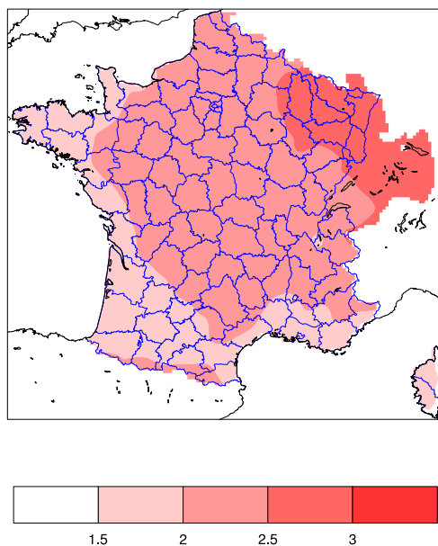
FIGURE 13 – Moyenne multi-modèles des anomalies de température (degrés C) pour la période hivernale (décembre-janvier-février (DJF)) couvrant 2046-2065 par rapport à la climatologie 1961-1990. Les modèles sont ceux du GIEC ainsi que les 7 simulations ARPEGE V4.
