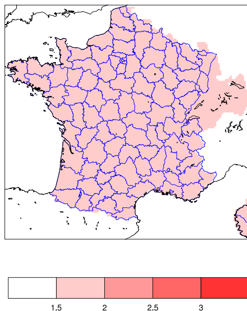
FIGURE 14 – Moyenne multi-modèles des anomalies de température (degrés C) pour la période estivale (juin-juillet-août (JJA)) couvrant 2046-2065 par rapport à la climatologie 1961-1990. Les modèles sont ceux du GIEC ainsi que les 7 simulations ARPEGE V4.
