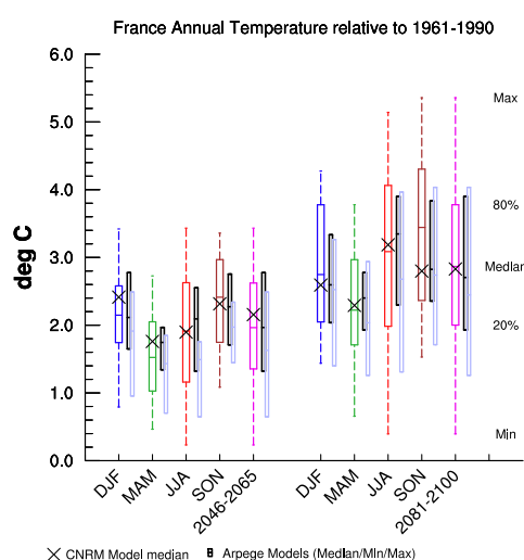
FIGURE 9 – Diagramme en boîte de l'anomalie de température pour les périodes 2046-2065 et 2081-2100 avec comme période de référence 1961-1990. Les boîtes de couleurs représentent la moyenne des simulation GIEC, les noires représentent les 4 simulations ARPEGE V4 CERFACS, et les boîtes violettes représentent les 3 simulations ARPEGE V4 RETIC. Le symbole X présente la simulation du modèle CNRM-CM3 de Météo-France. Les boîtes noires et violettes ne présentent que les extrêmes maximum et minimum de même que la médiane (pas de lignes tiretées). La moyenne spatiale est calculée sur un domaine couvrant la France entière.
